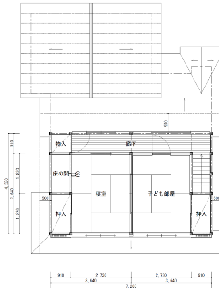
2階平面図
