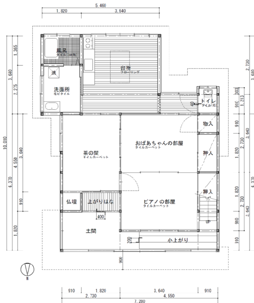
1階平面図
